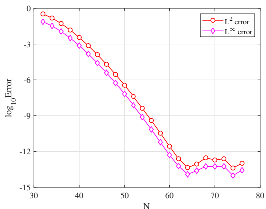
图 5.3 谱方法的误差.
