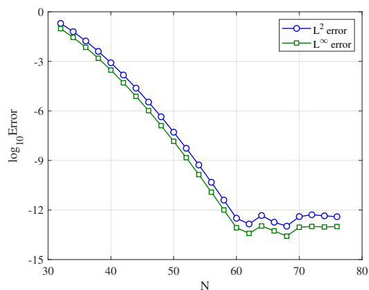
图 5.4 配置方法的误差.
